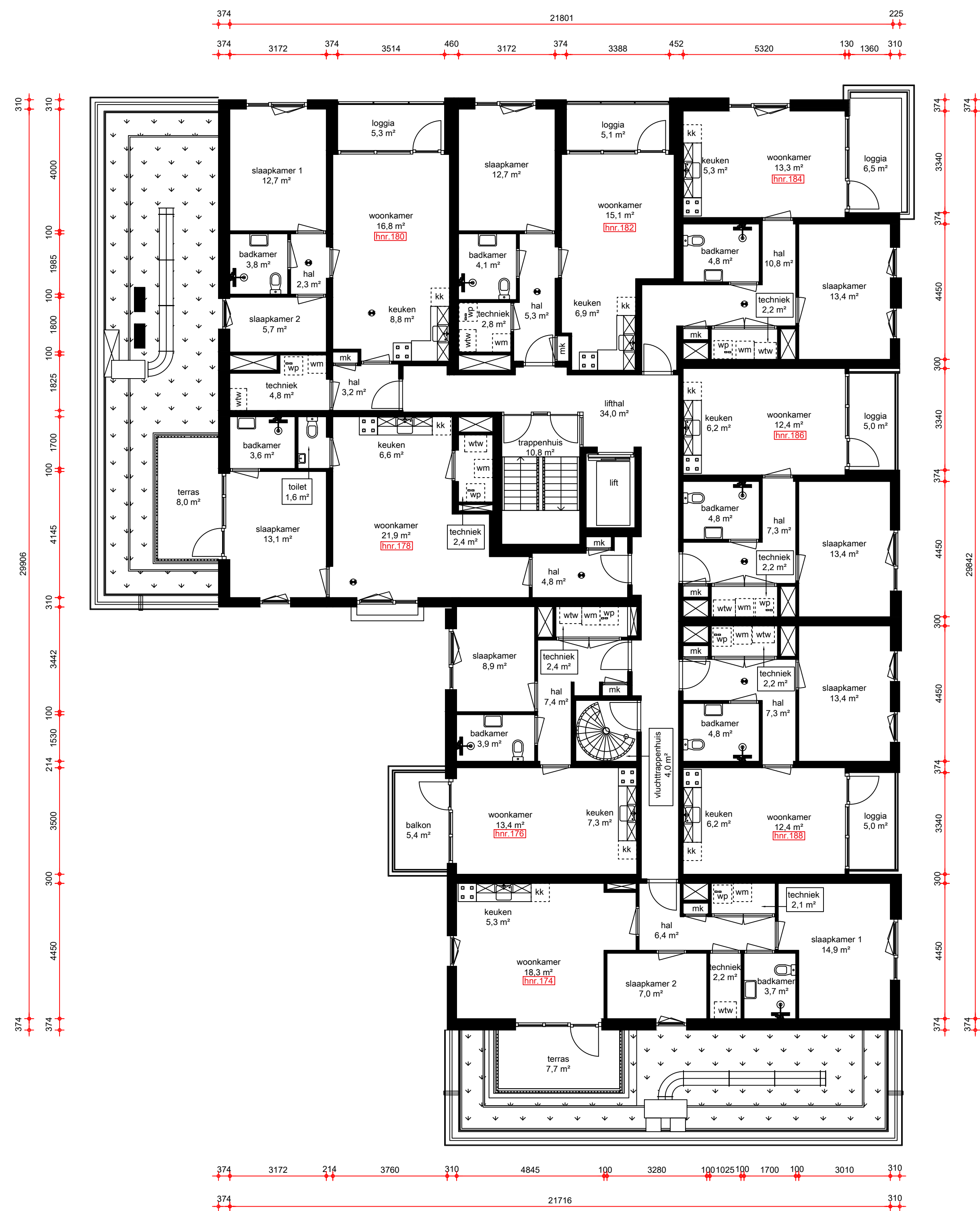
derde verdieping
